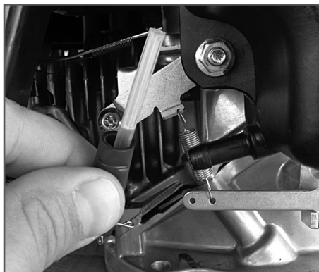
Рис. 11 Топливный фильтр
