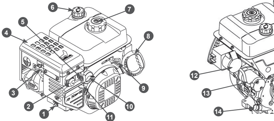
Рис. 3. Основные узлы и органы управления двигателя
