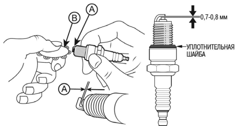
Рис. 38. Проверка межэлектродного зазора А – зазор В – щуп
