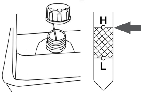
Рис. 23. Проверка уровня масла по щупу верхней маслозаливной горловины
