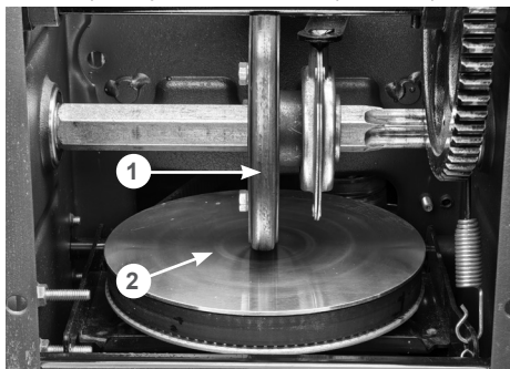
Рис. 13. Проверка нейтрального положения фрикционного колеса
