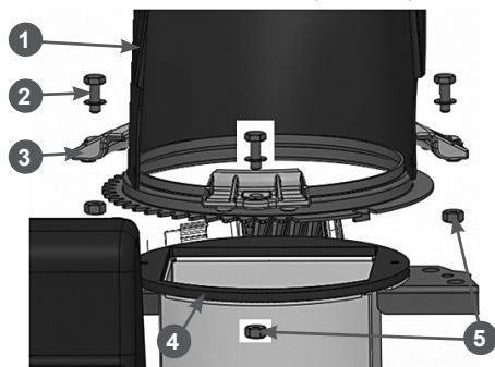
Рис. 15. Установка жёлоба выброса снега
