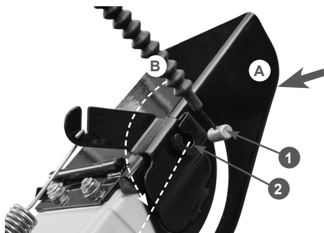
Рис. 16. Установка наконечника троса управления дефлектором жёлоба
