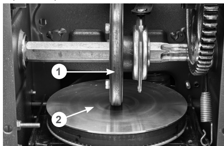
Рис. 41. Обслуживание трансмиссии
