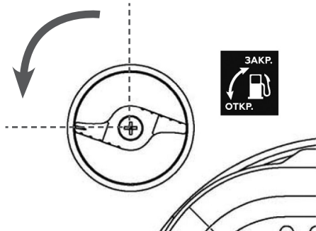
Рис. 26. Рычаг топливного крана
