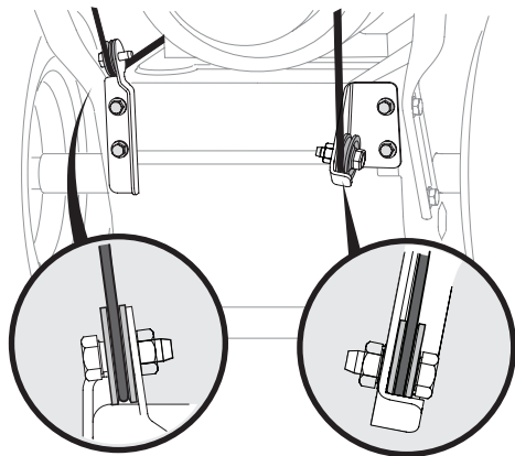
Рис. 6. Положение тросов на роликах
