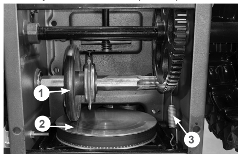
Рис. 9. Проверка регулировки троса включения хода
