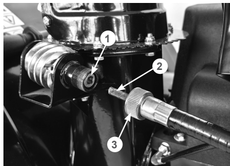
Рис. 18. Подсоединение гибкого вала к червячному валу
