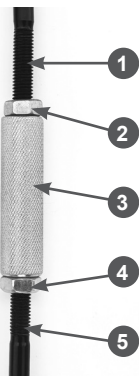
Рис. 14. Регулировка длины тяги рычага переключения передач
