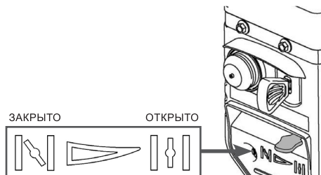
Рис. 29. Рычаг управления воздушной заслонкой
