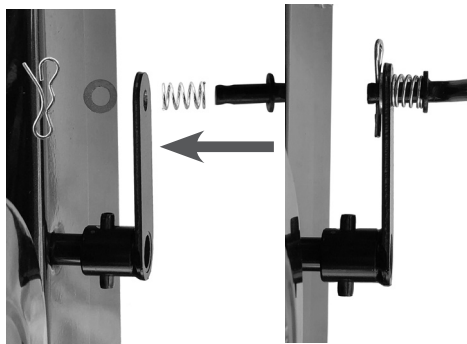
Рис. 11. Подключение тяги к нижнему рычагу
