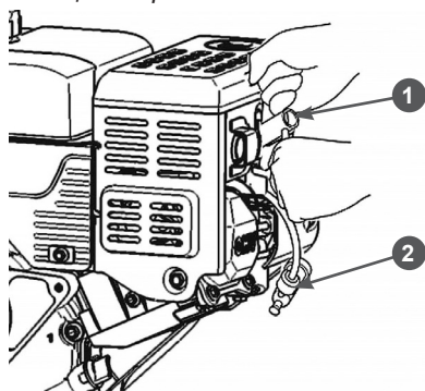
Рис. 37. Обслуживание свечи зажигания
