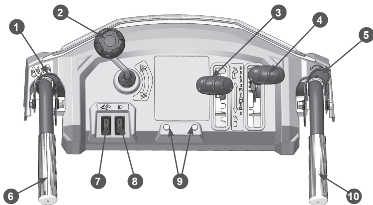
Рис. 2. Панель управления (вид со стороны оператора)
