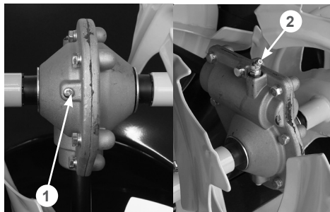
Рис. 39. Добавление смазки в редуктор
