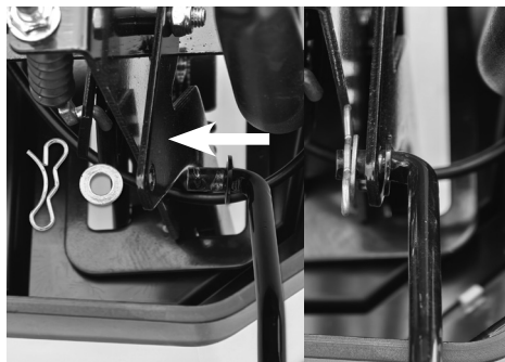
Рис. 10. Подключение тяги к рычагу переключения передач
