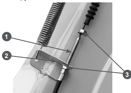
Рис. 17. Установка оболочки троса управления дефлектором жёлоба
