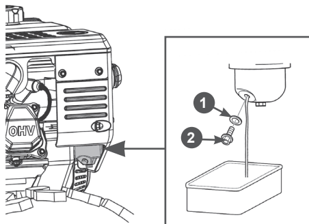
Рис. 36. Слив топлива с карбюратора
